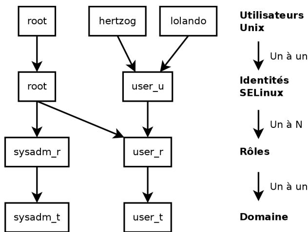
FIGURE 14.3 Contextes de sécurité et utilisateurs Unix
