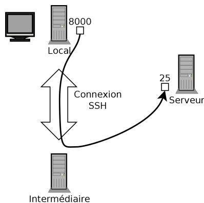
FIGURE 9.3 Déport d’un port local par SSH
