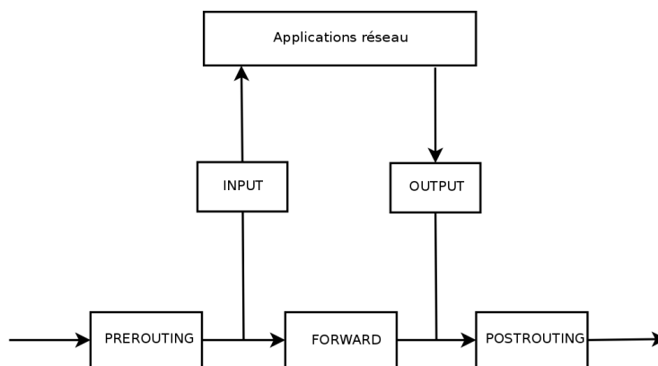
FIGURE 14.1 Ordre d'emploi des chaînes de netfilter
