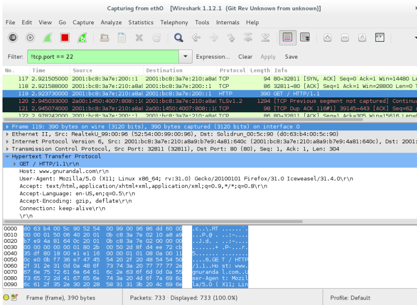
FIGURE 10.1 Analyseur de trafic réseau wireshark
