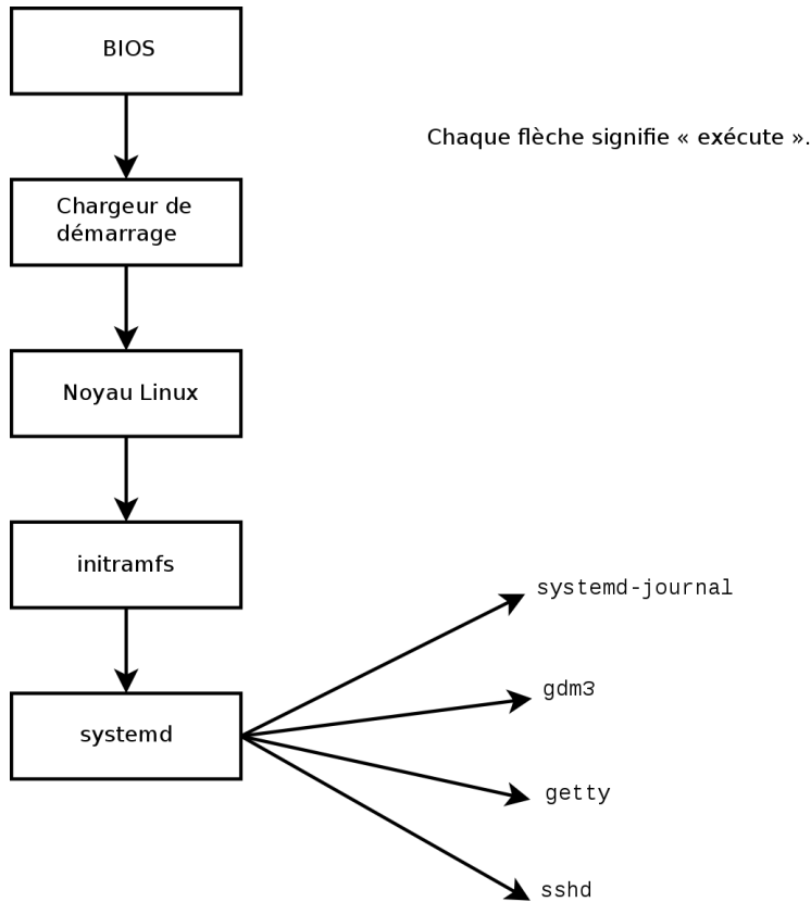
FIGURE 9.1 Étapes du démarrage d’un ordinateur sous Linux avec systemd
