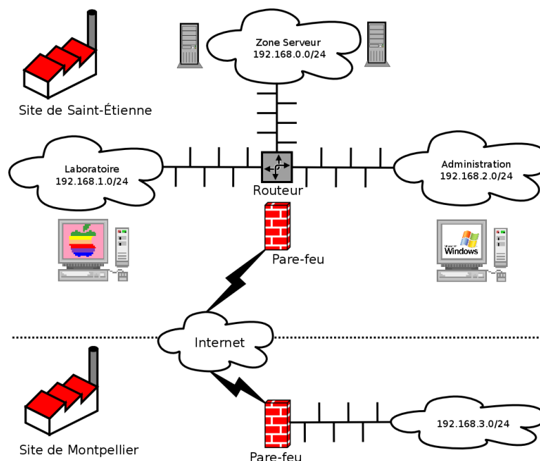
FIGURE 2.1 Aperçu global du réseau de Falcot SA
