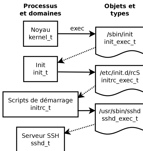
FIGURE 14.4 Transitions automatiques entre domaines
