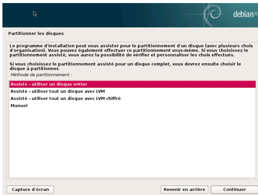
FIGURE 4.7 Choix du mode de partitionnement
