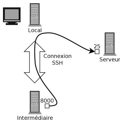
FIGURE 9.4 Déport d’un port distant par SSH
