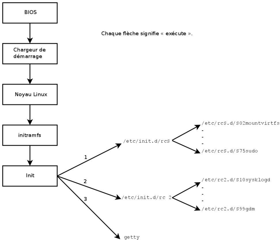
FIGURE 9.2 Étapes du démarrage d'un ordinateur sous Linux avec le système d'initialisation System V
