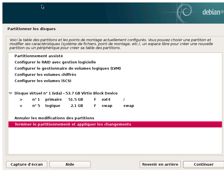
FIGURE 4.10 Valider le partitionnement
